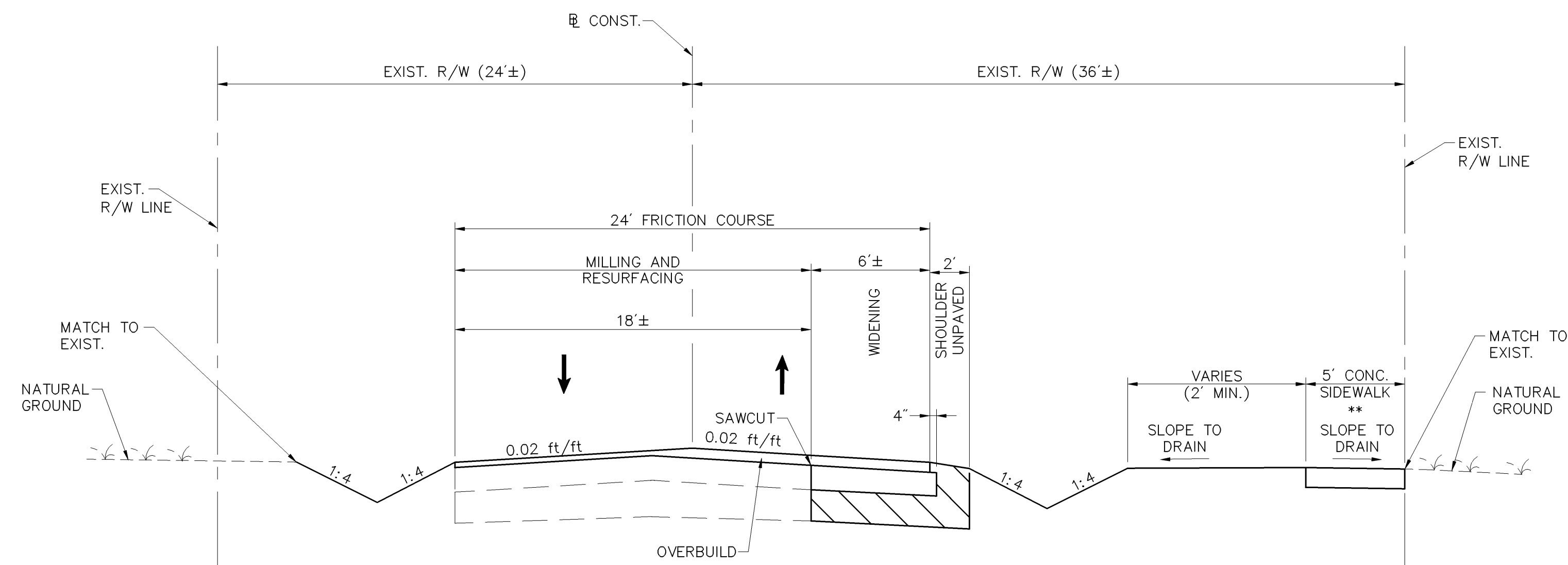
TYPICAL SECTION 02 N.T.S.
