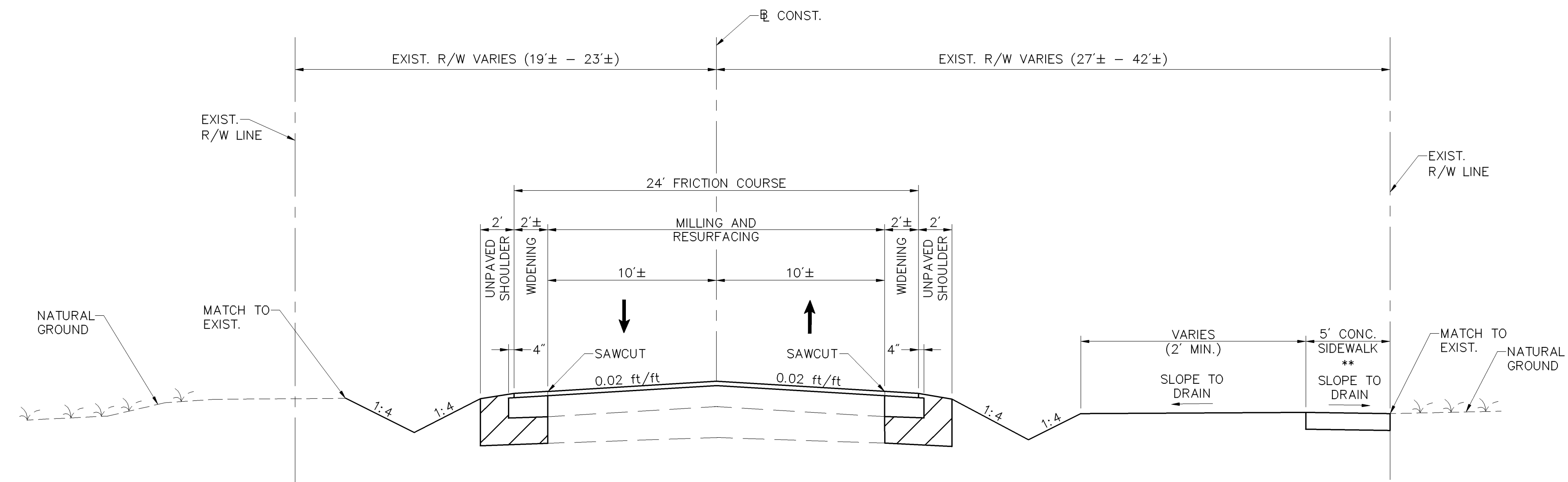
TYPICAL SECTION 01 N.T.S.
